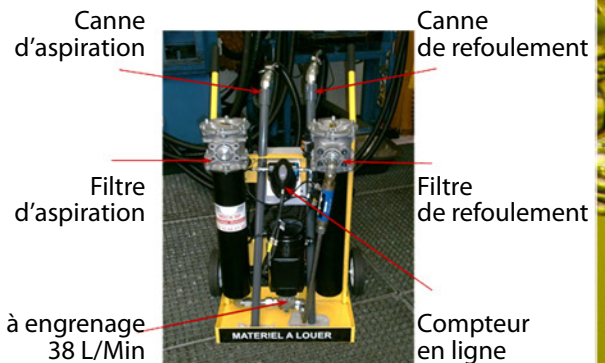
Principe de circulation
